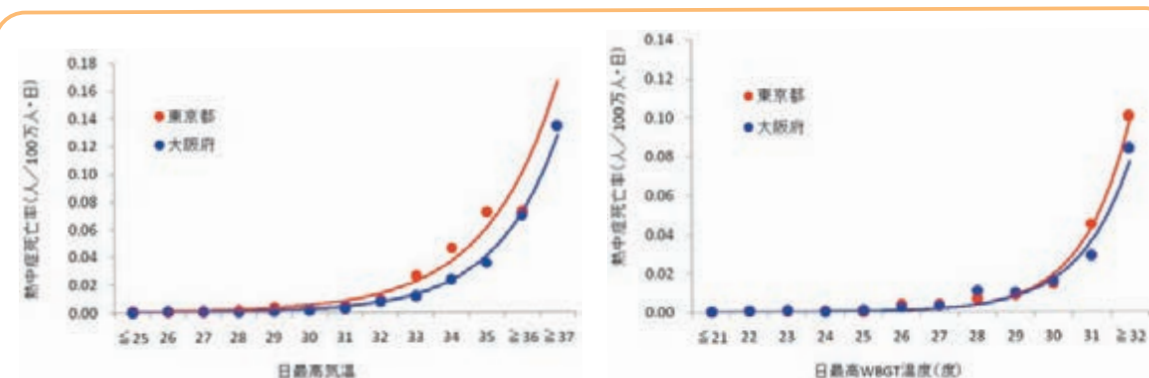
図1-11 日最高気温別熱中症死亡率と日最高暑さ指数(WBGT)別熱中症死亡率(1972~1996年)
