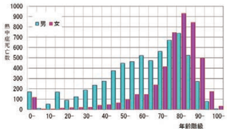
図1-7 熱中症死亡数の年齢階級別累積(1968年~2012年)
