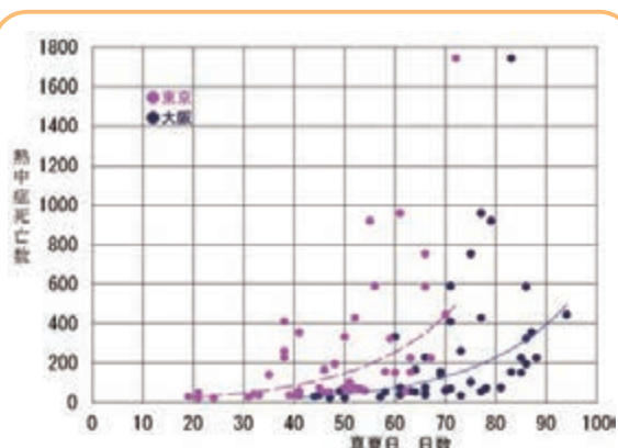
図1-9 熱中症死亡数と真夏日日数の関係(1968~2012年)
