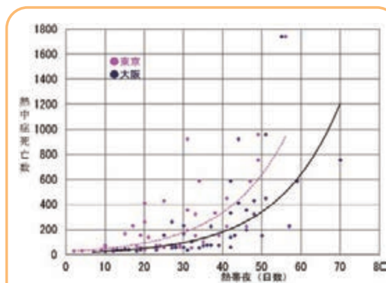
図1-10 熱中症死亡数と熱帯夜日数の関係(1968~2012年)
